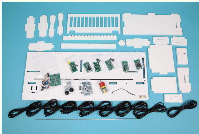
Maquette livrée en kit : BE-APORT-COUL-KIT
